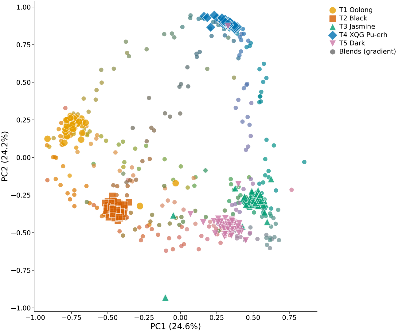
CARL — PCA (25%+24%)
