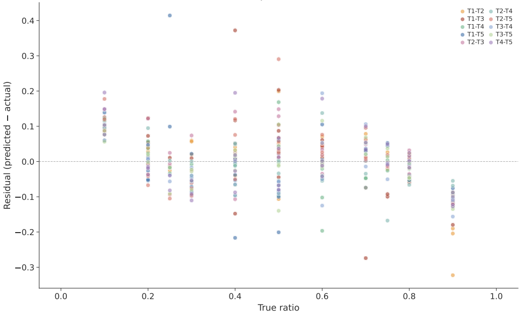
CARL-Proj + SVR residuals
