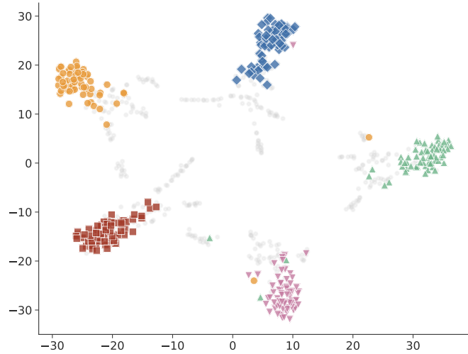
t-SNE (HC)
