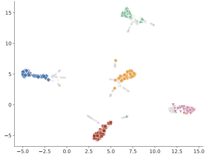
UMAP (HC)
