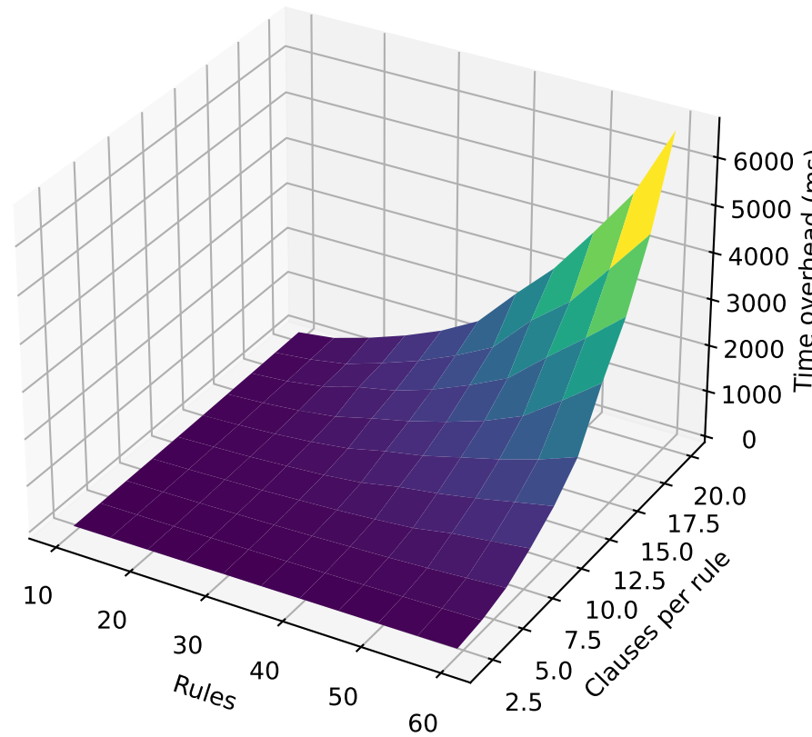
ASMETA Server
