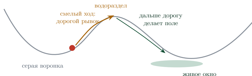
Рис. 13: Рельеф судьбы: два водосбора и гребень между ними. До гребня — каждый шаг дорог; за гребнем тот же закон несёт сам. Смелость — плата за пересечение водораздела, и в естественной мере расстояний она совпадает с кратчайшим путём: навигатор, ищущий кратчайшее, переоткрывает смелость (машинно проверено).
