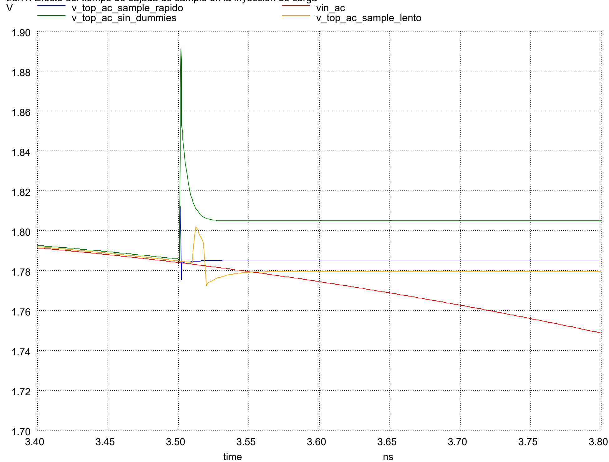
tran1: Efecto del tiempo de bajada de sample en la inyeccion de carga
