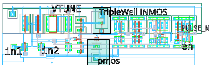
Figura 3.4: Generator de pulso con nmos de triple-well
