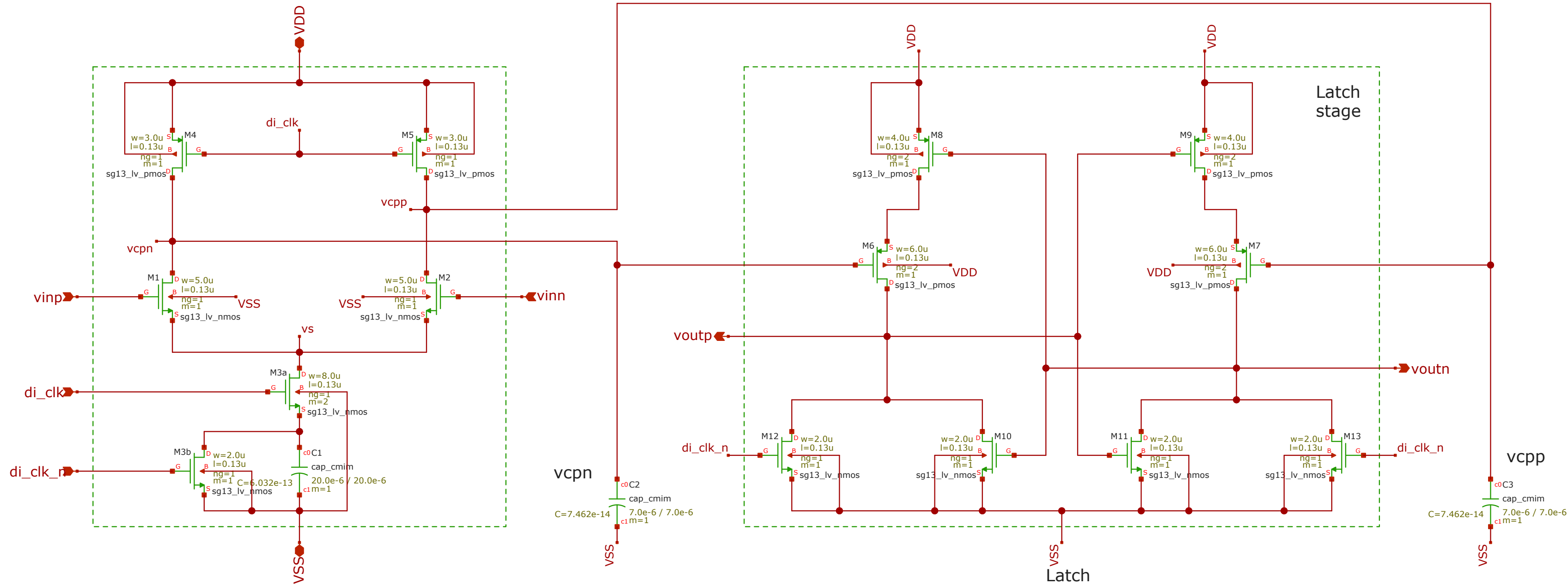
PreAmp con capacitor de cola
