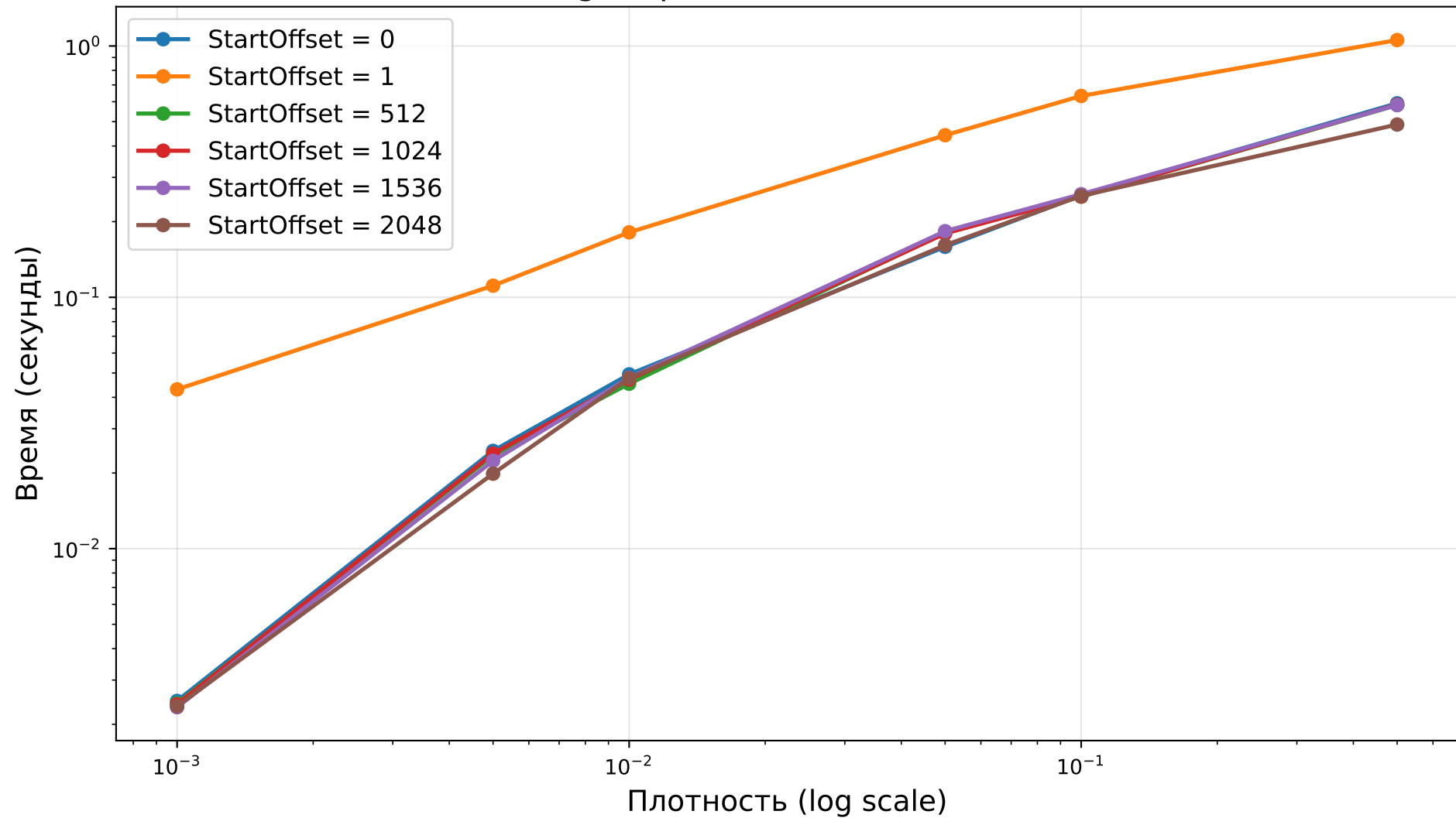
MatrixSliceAlign: время vs плотность (Size = 4096)
