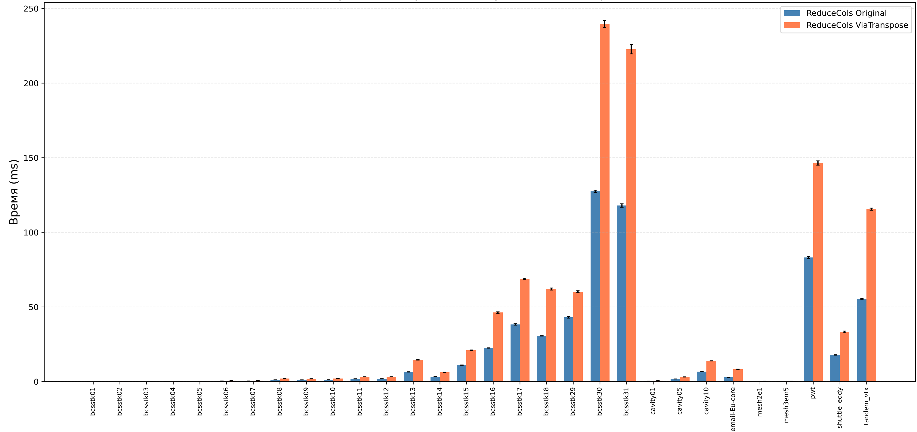
Сравнение времени: Original vs ViaTranspose
