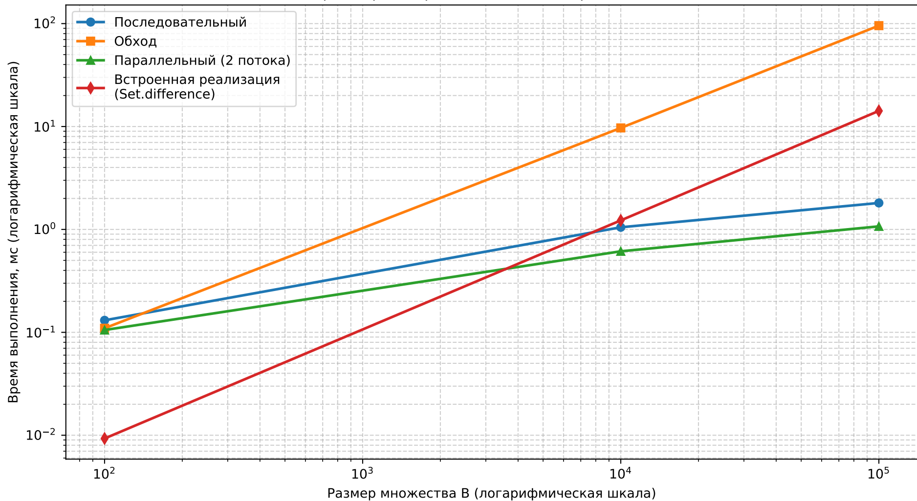
Зависимость времени выполнения операции разности от размера второго множества (при A = 1000 )
