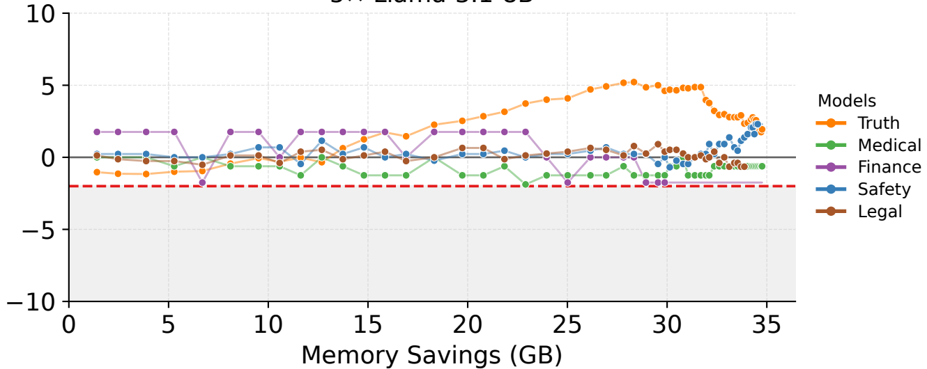
5x Llama-3.1-8B
