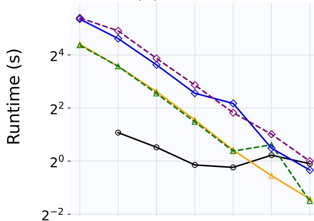
(d) GAP-urand
