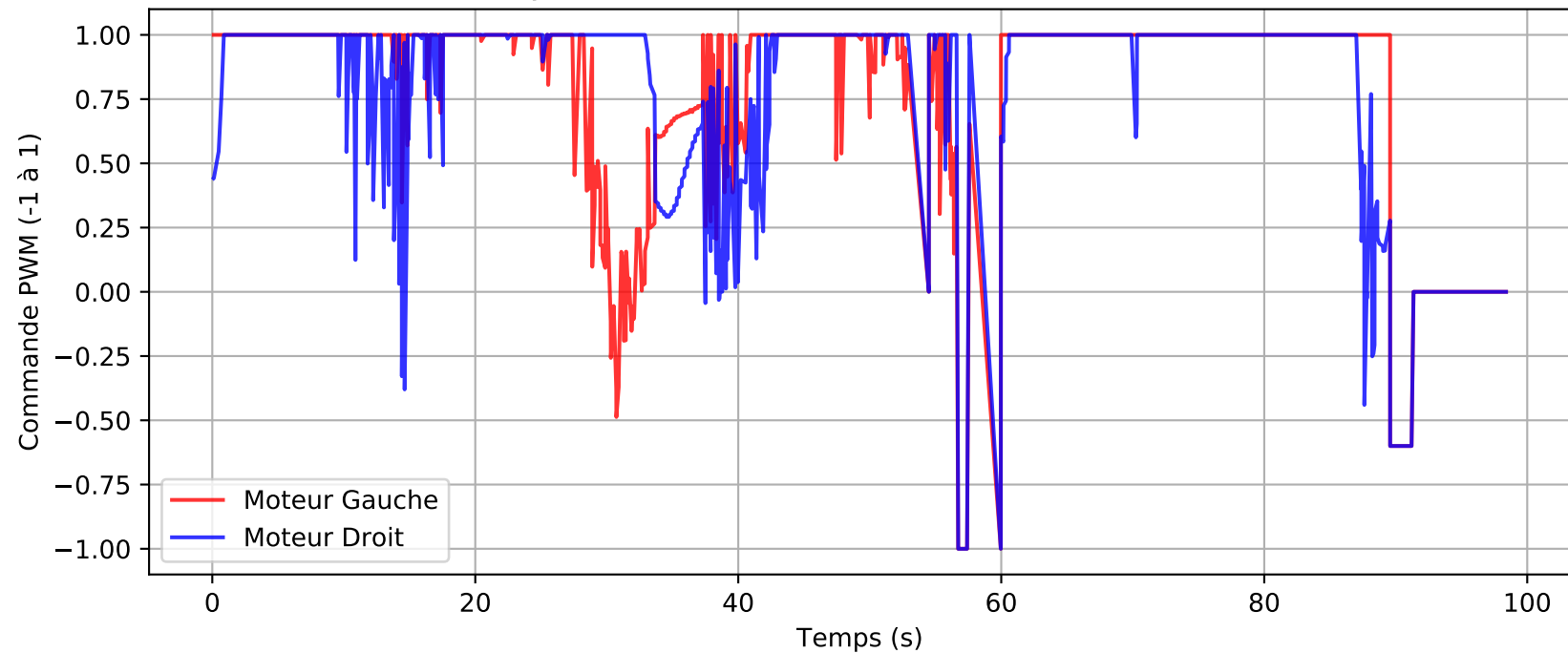
Test 1 - Sanity Check (Chicane) : Profil des Commandes (RL + Shield)
