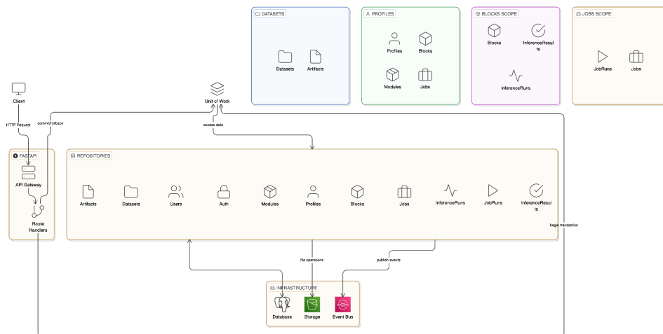
Figura 9 – Diagrama de alto nível da arquitetura do back-end.
