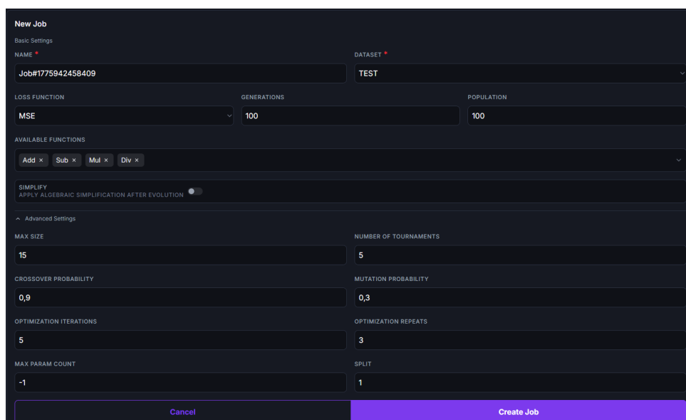
Figura 24 – Tela de configuração de um novo Job na plataforma Spectrum, onde os usuários podem configurar os meta-parâmetros do algoritmo eggp, como o número de gerações, o tamanho da população e as funções a serem utilizadas, entre outros
