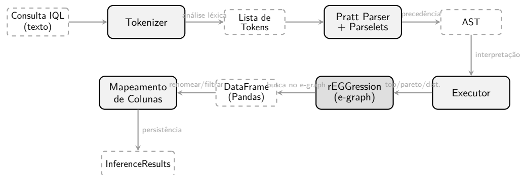
Figura 29 – Pipeline de execução de uma consulta IQL, desde a entrada textual do usuário até o armazenamento dos resultados como InferenceResults no banco de dados
