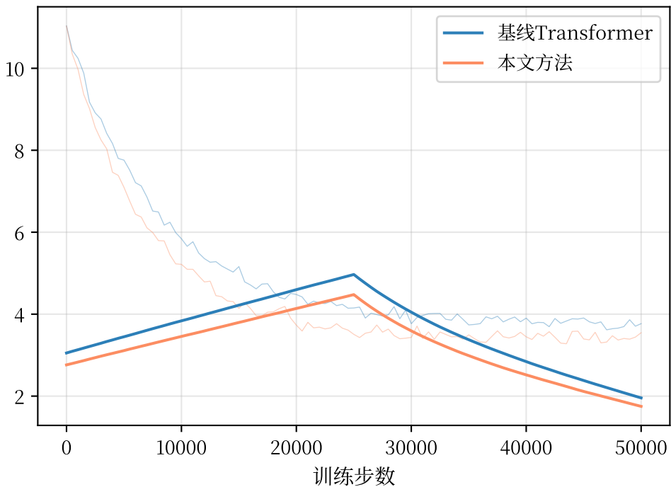
交叉熵损失
