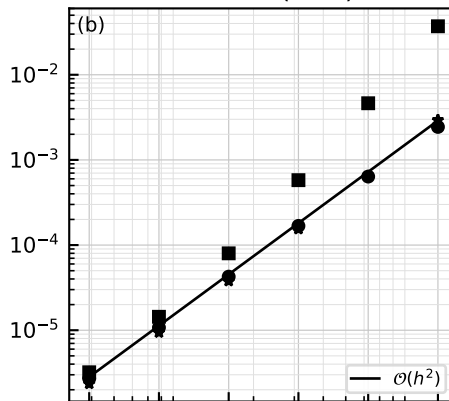
Smooth (k=2)
