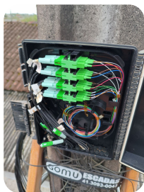
Foto da Caixa (CEO/CTO/BOX...)
