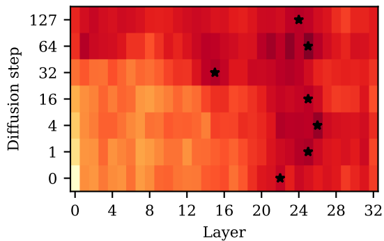
LLaDA-8B / JSON Schema
