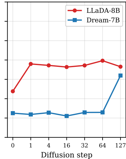
ARC
