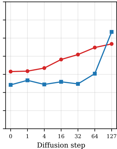
GSM8K
