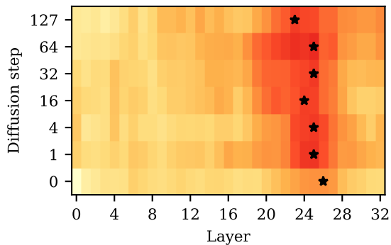
LLaDA-8B / ARC
