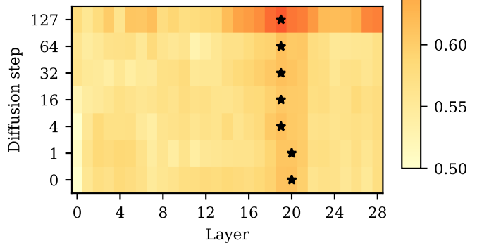
Dream-7B / ARC
