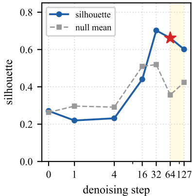
LLaDA mbpp (code)
