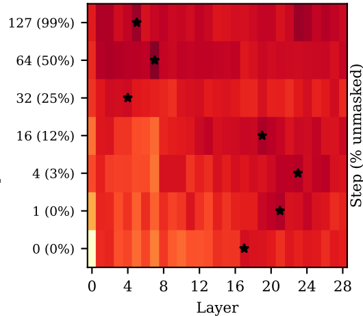
Dream-7B / JSON Schema
