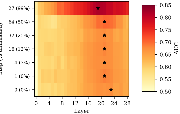
Dream-7B / GSM8K
