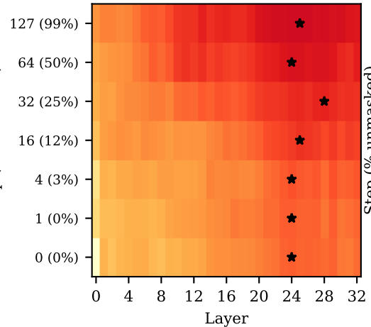
LLaDA-8B / GSM8K
