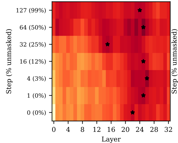
LLaDA-8B / JSON Schema
