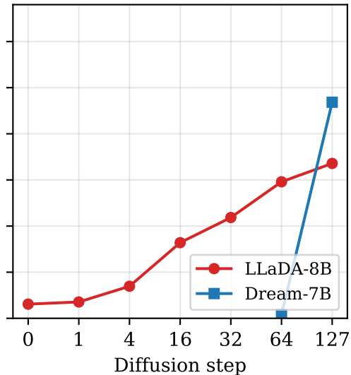
GSM8K
