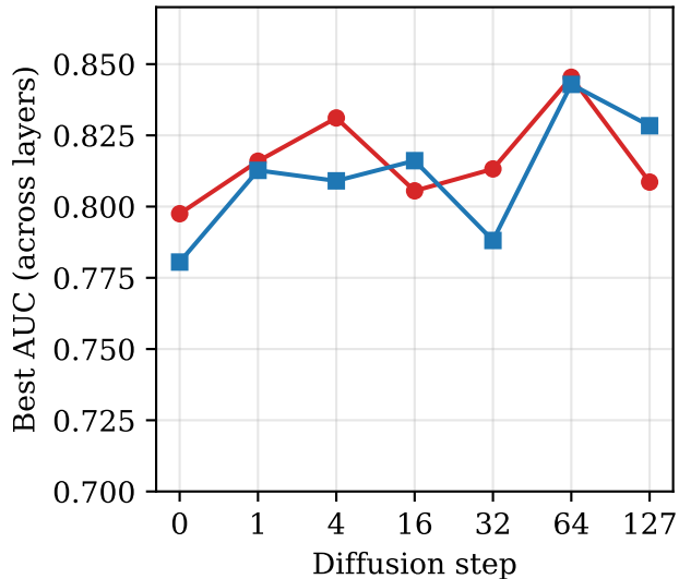
JSON Schema
