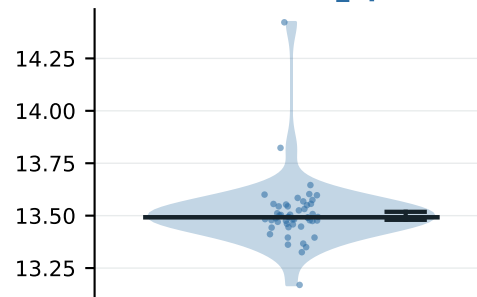
DaCe auto_opt
