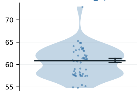
DaCe auto_opt
