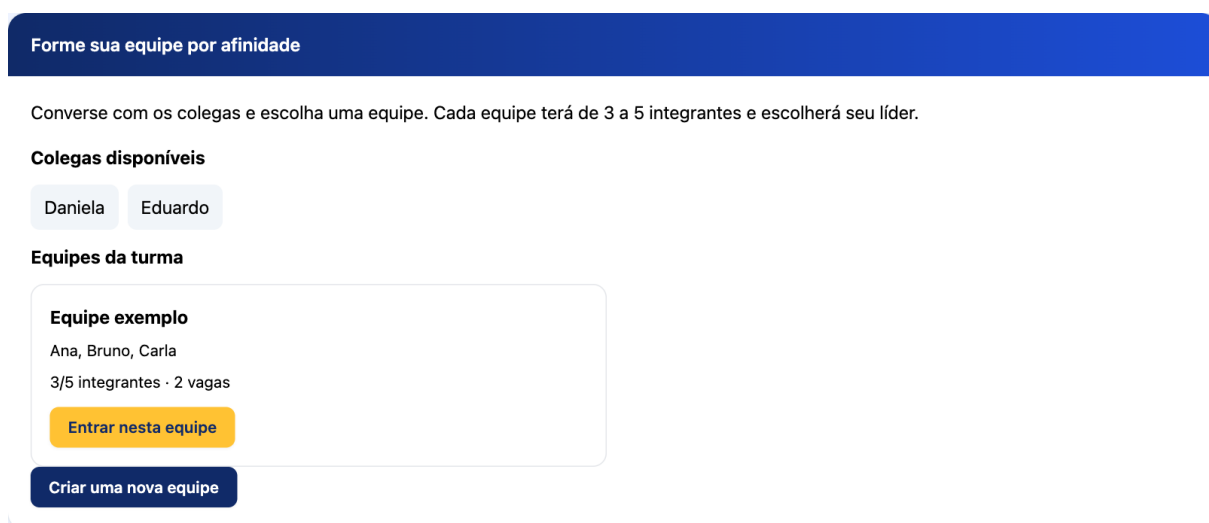
Figura 3 - Tela de colegas e equipes
