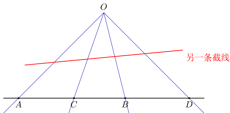
图 1: 同一四线束被不同截线所截, 所得四点交比不变
