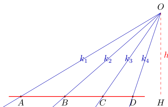
图 2: 调和线束的斜率模型
