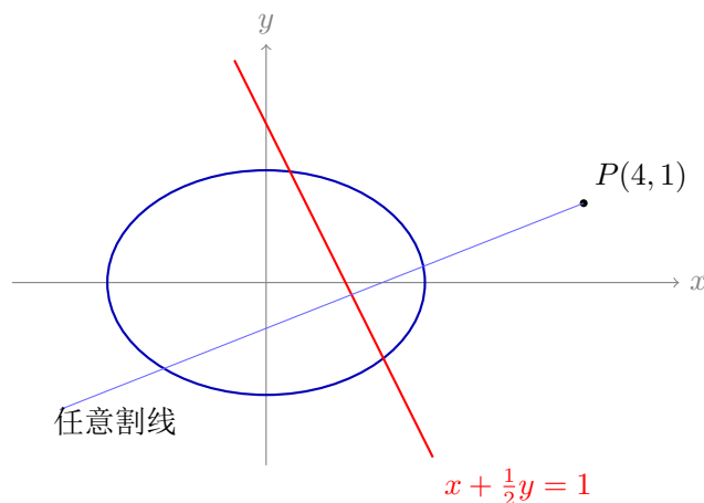
图 3: 割线上的调和共轭点落在固定极线上
