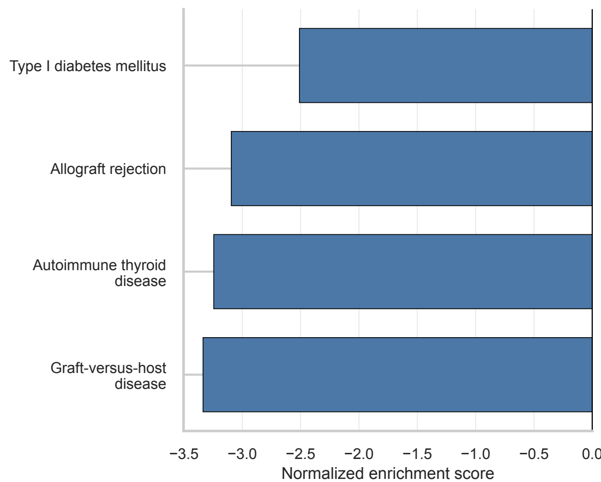
KEGG
