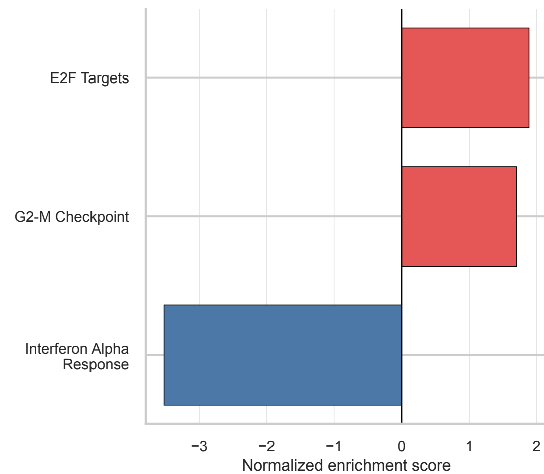
MSigDB Hallmark
