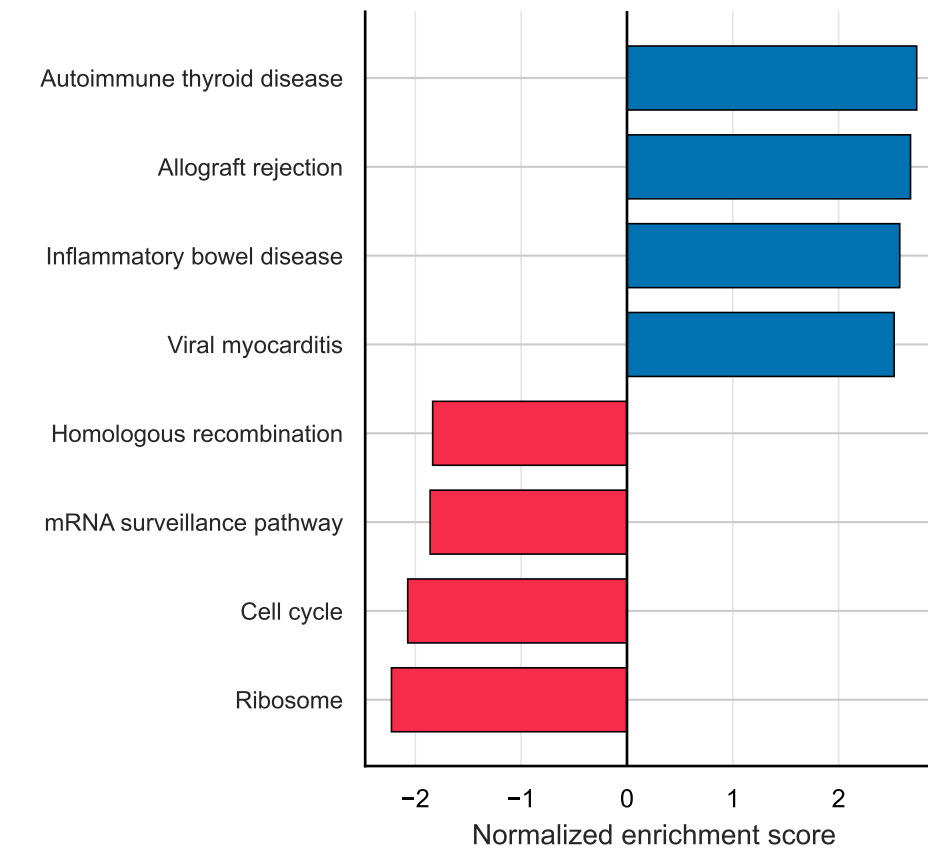
Lung: KEGG
