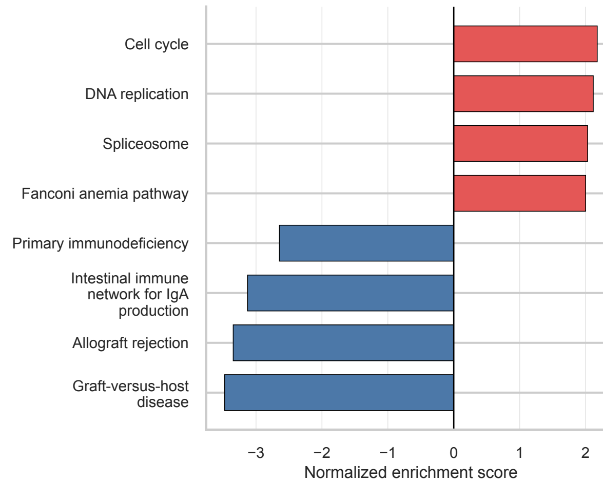
KEGG
