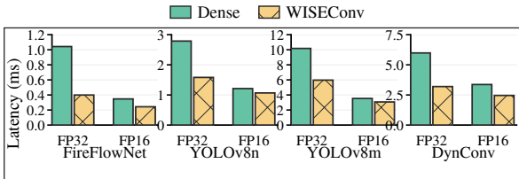
(a) RTX 3080
