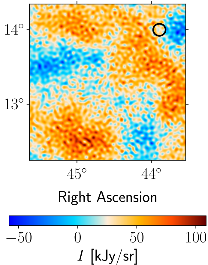
Data: Planck 100 GHz
