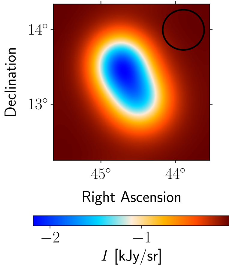
Model: Planck 30 GHz
