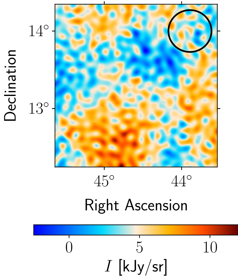
Data: Planck 30 GHz
