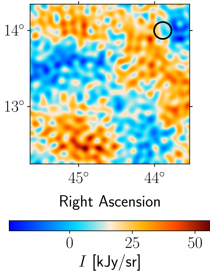
Data: Planck 70 GHz
