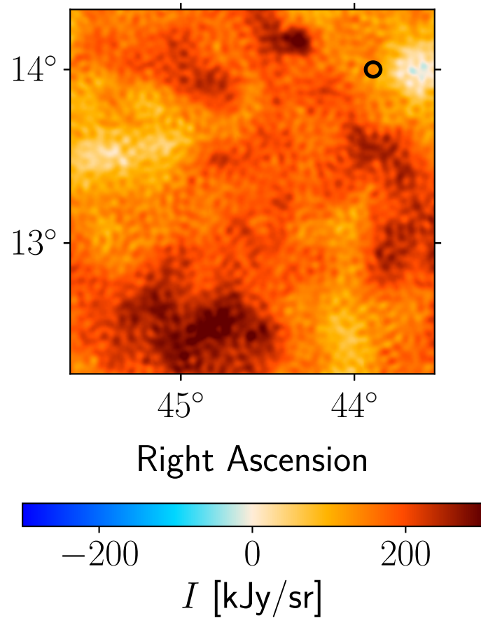
Data: Planck 217 GHz
