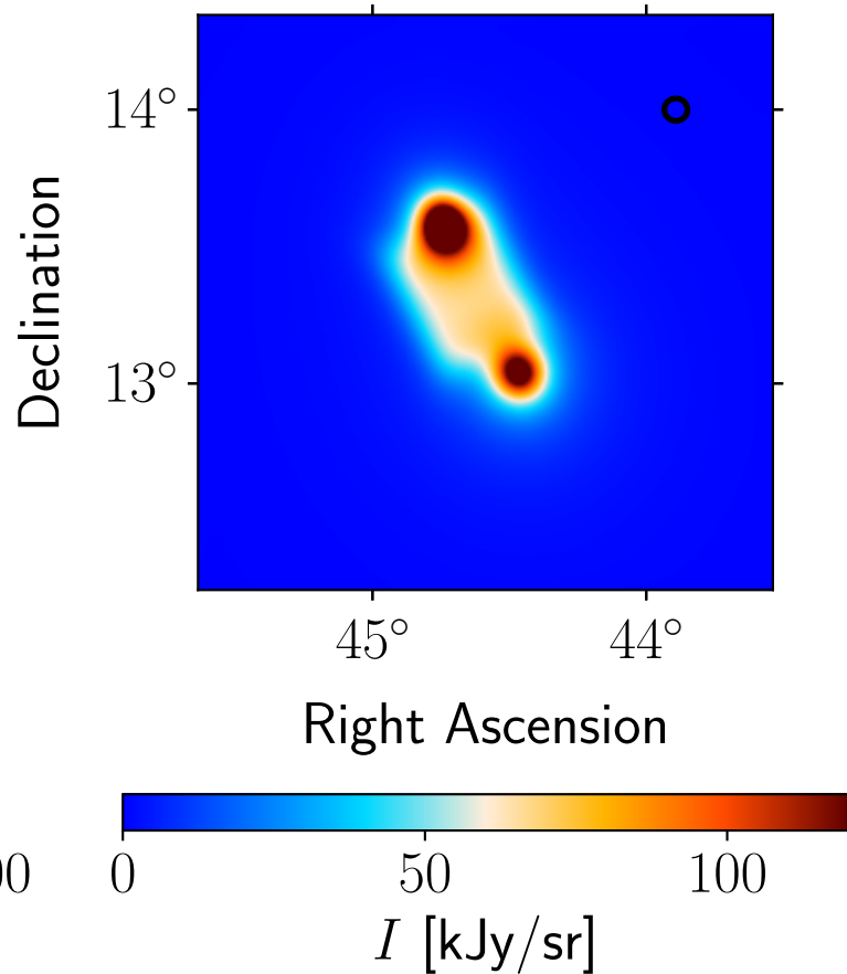
Model: Planck 353 GHz
