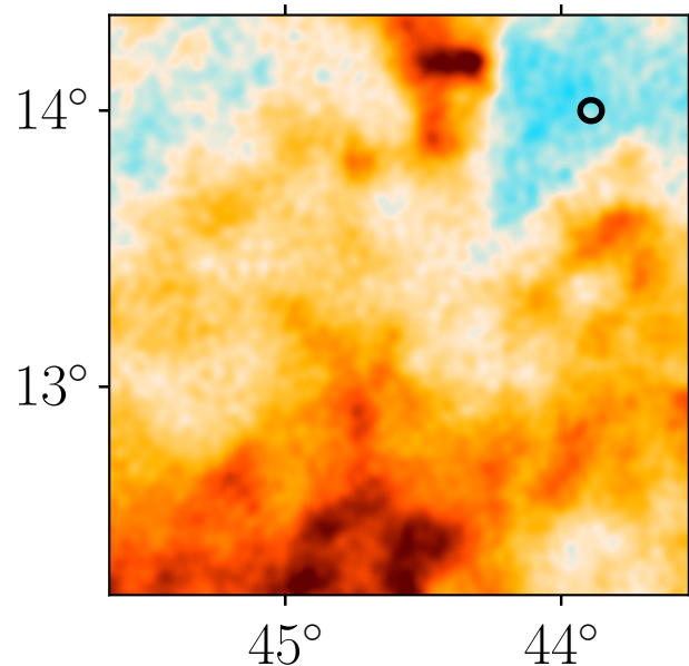
Data: Planck 545 GHz
