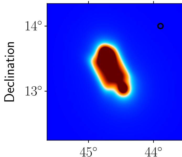
Model: Planck 545 GHz
