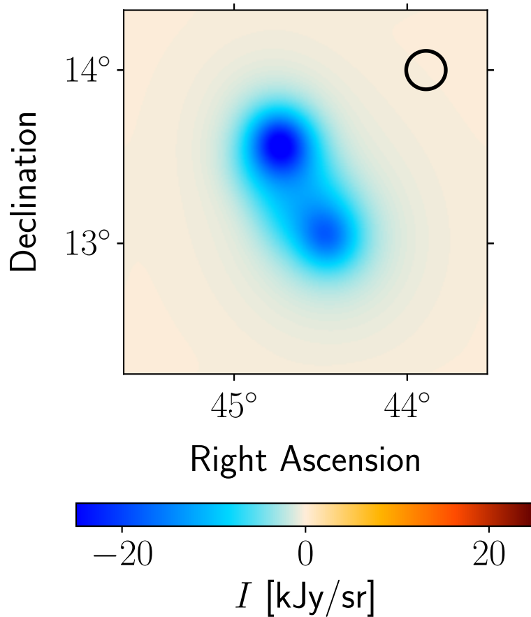
Model: Planck 70 GHz
