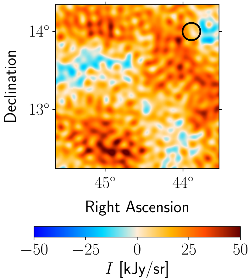
Data: Planck 70 GHz
