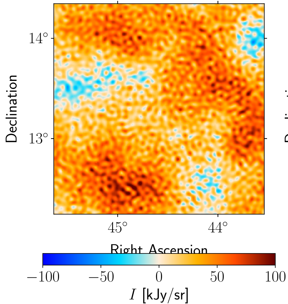
Data: Planck 100 GHz
