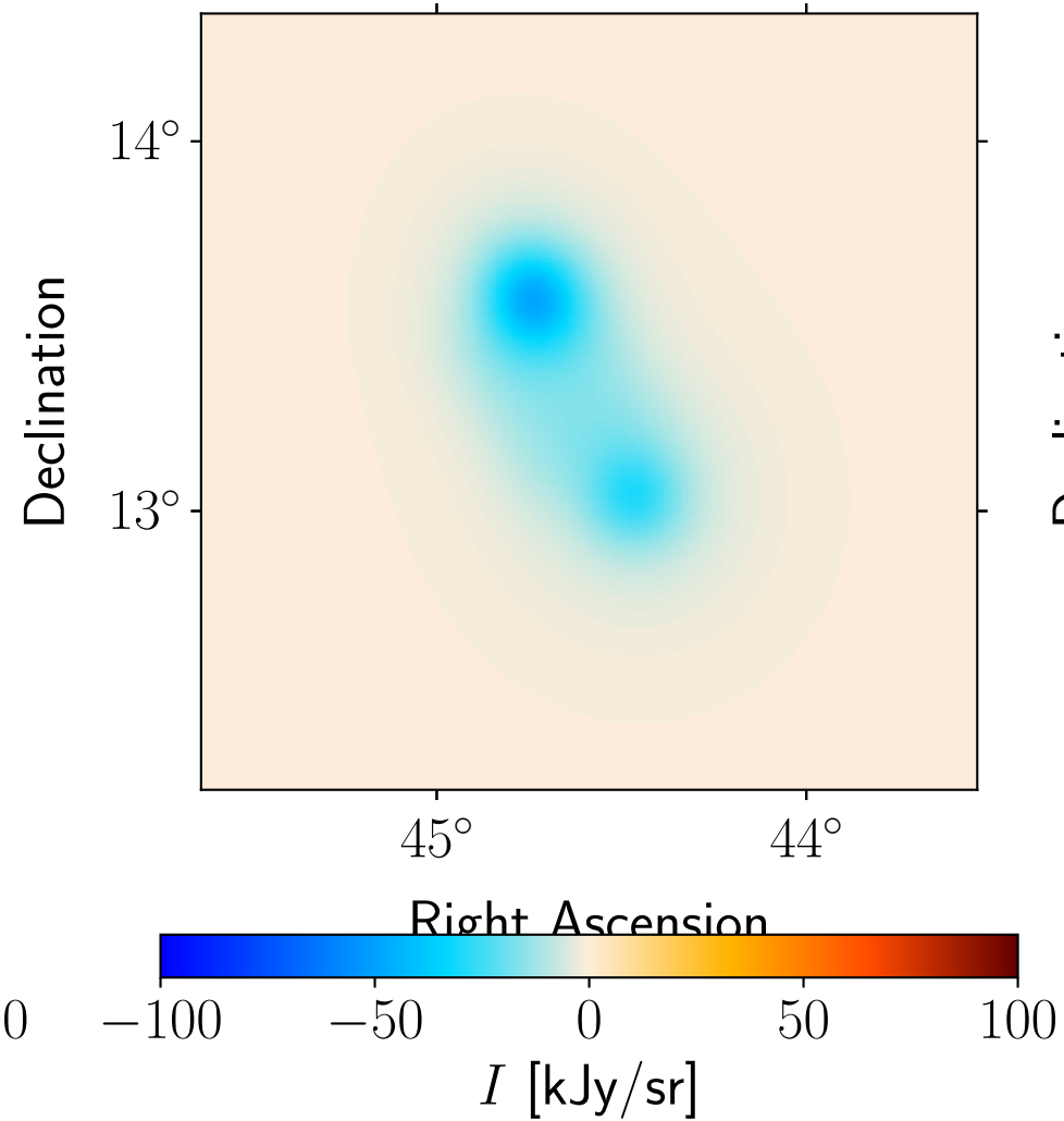
Model: Planck 100 GHz
