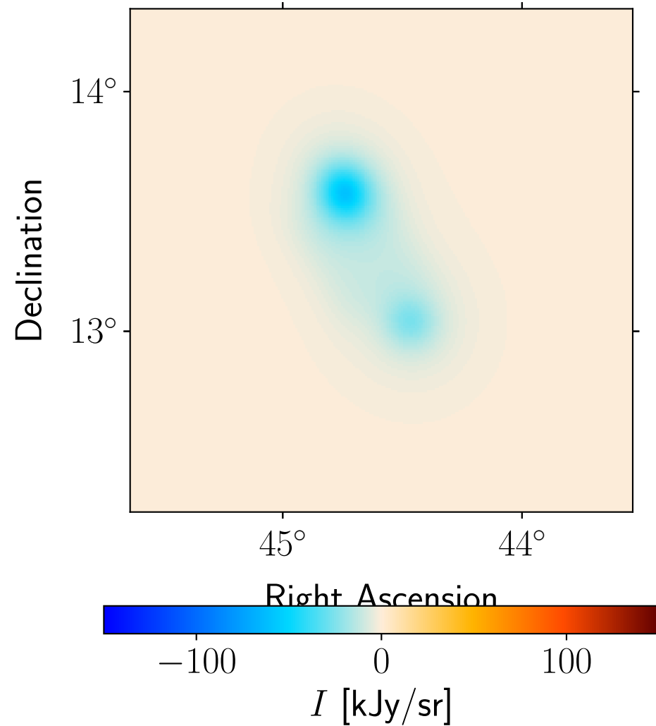
Model: Planck 143 GHz
