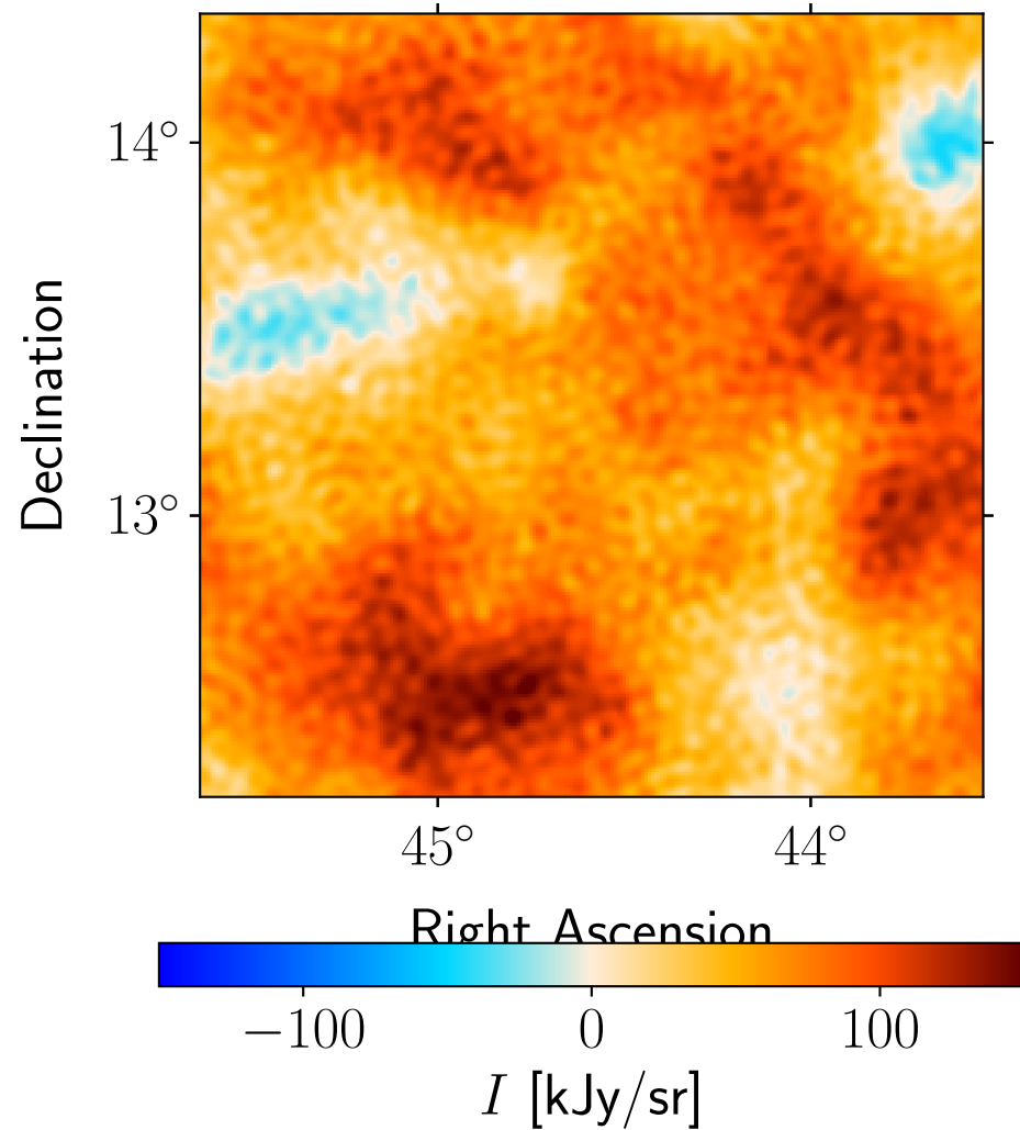
Data: Planck 143 GHz
