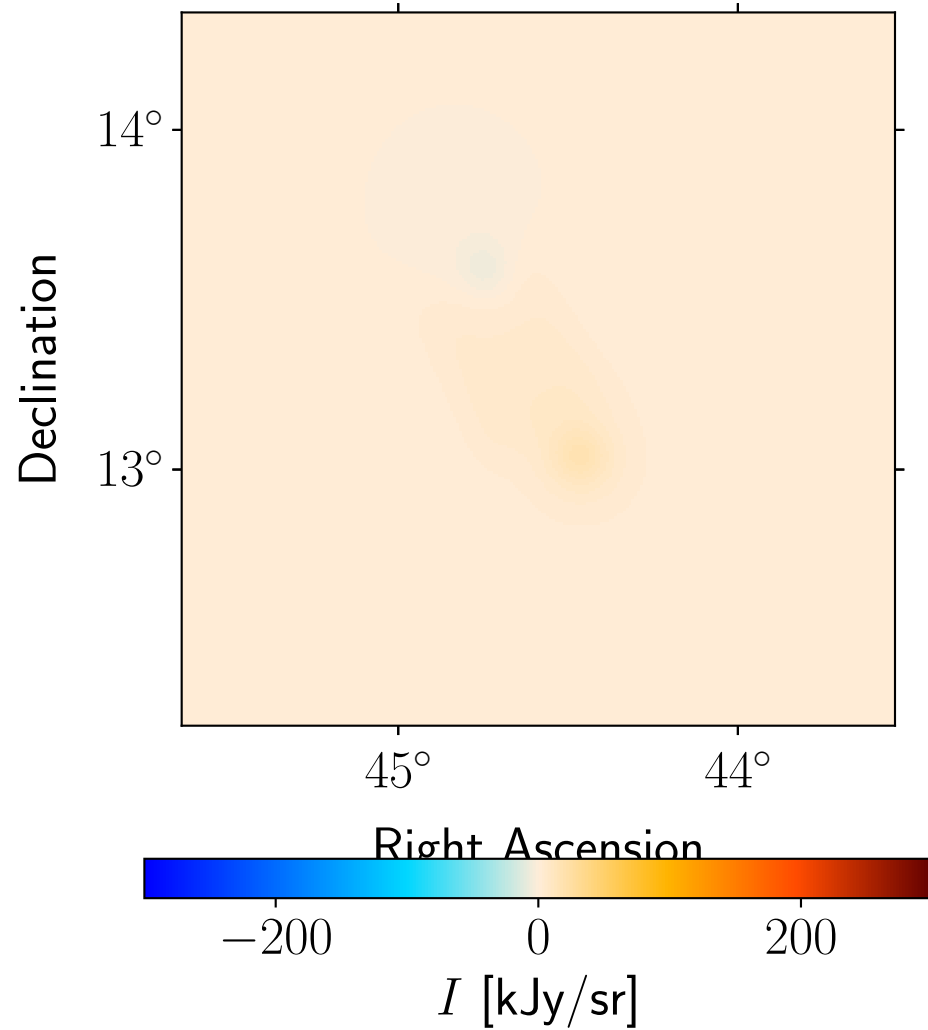
Model: Planck 217 GHz
