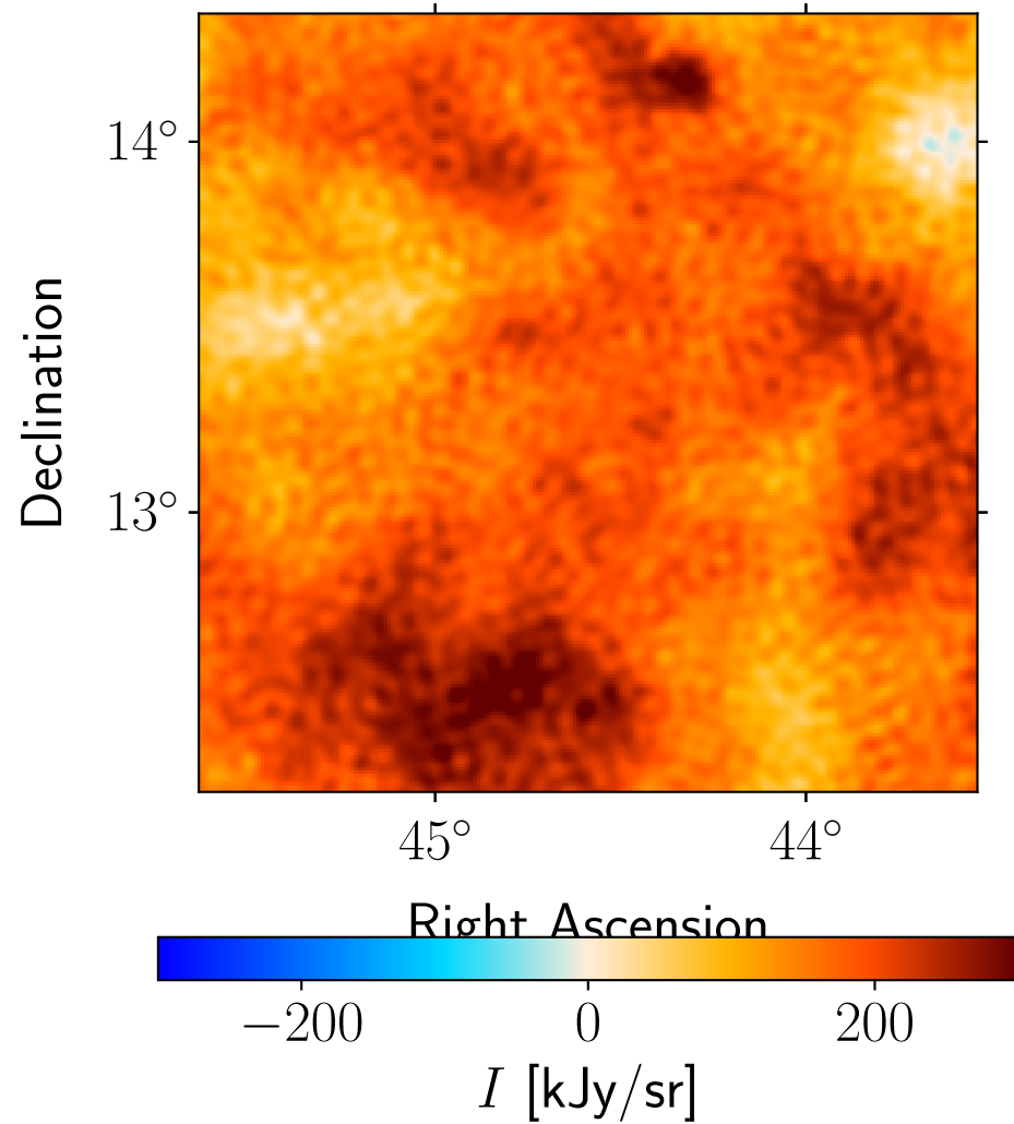
Data: Planck 217 GHz
