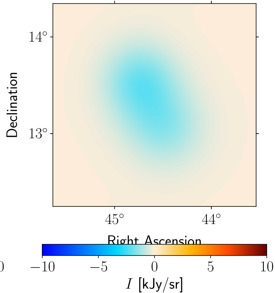
Model: Planck 30 GHz
