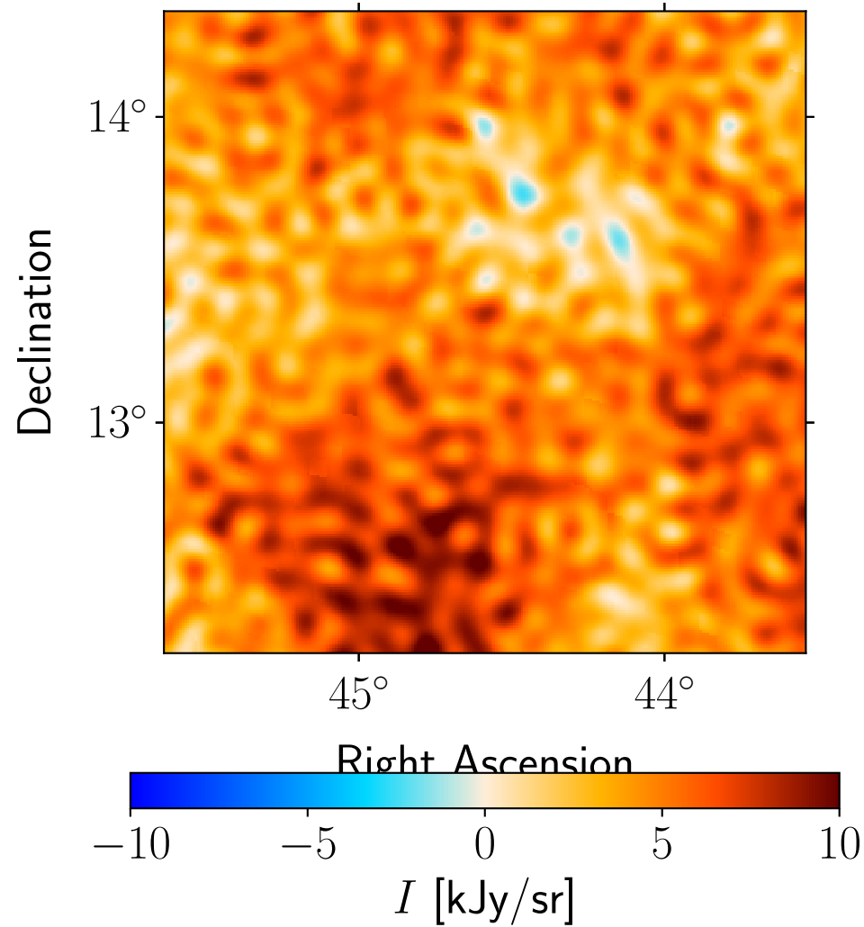
Data: Planck 30 GHz
