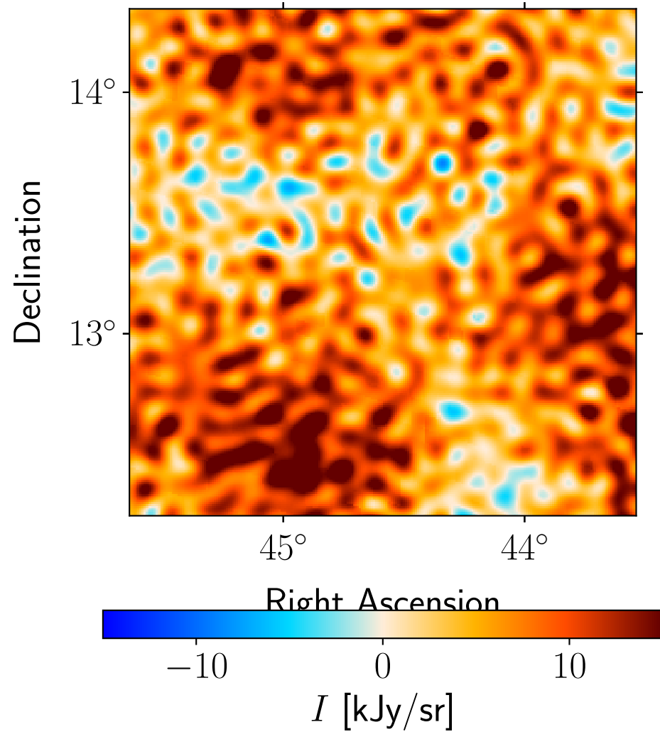
Data: Planck 44 GHz
