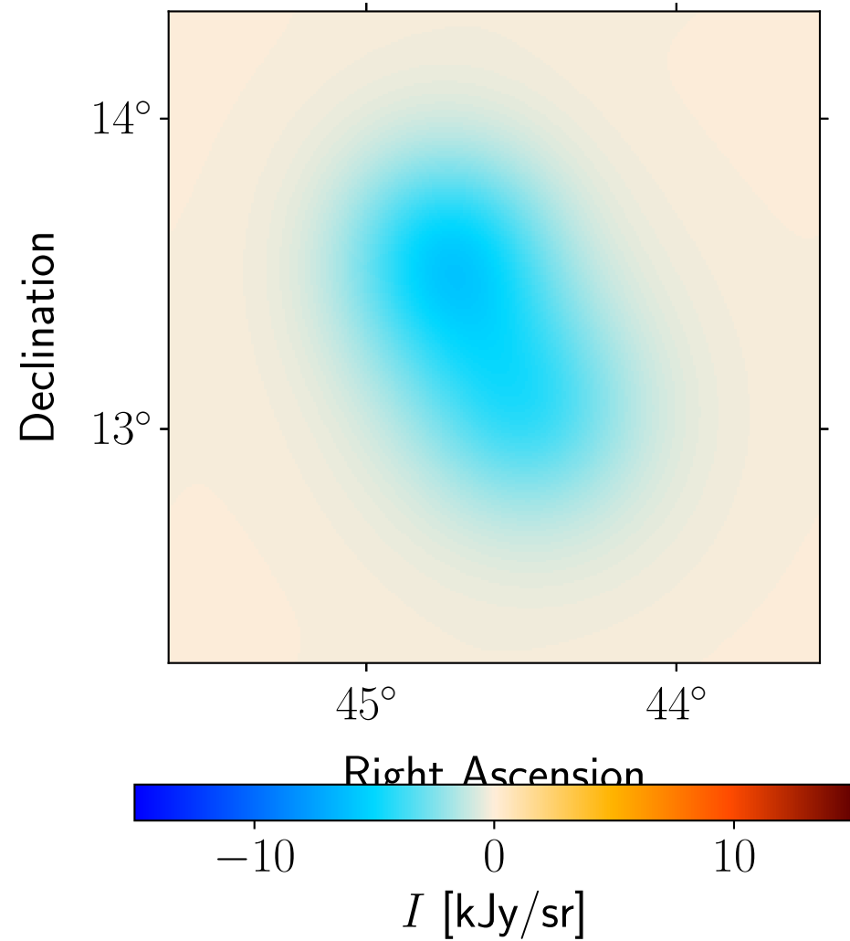
Model: Planck 44 GHz
