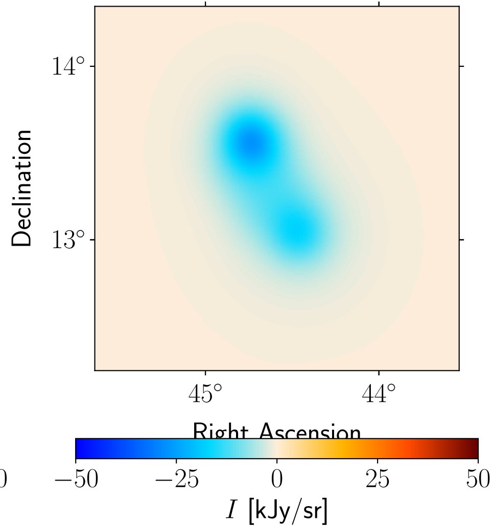
Model: Planck 70 GHz
