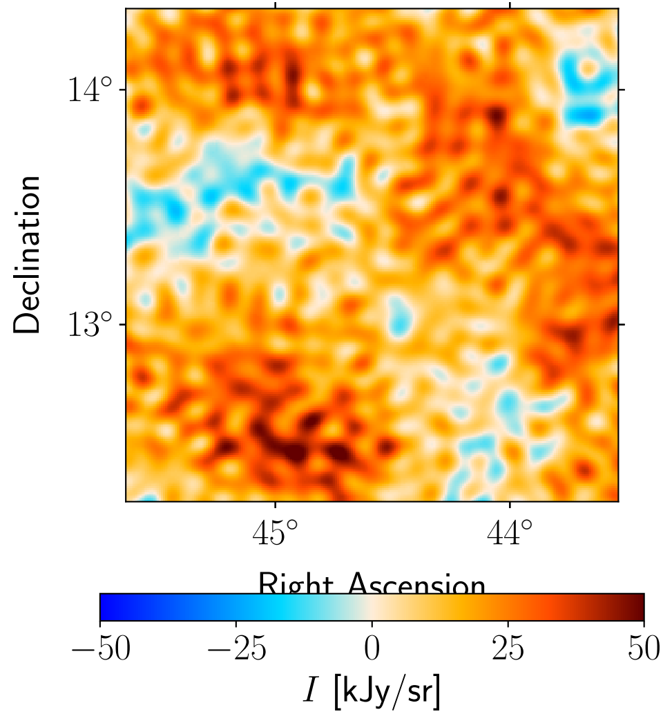
Data: Planck 70 GHz
