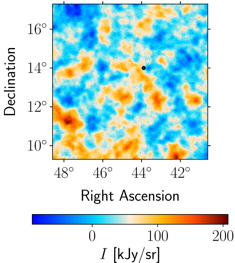
Data: Planck 143 GHz
