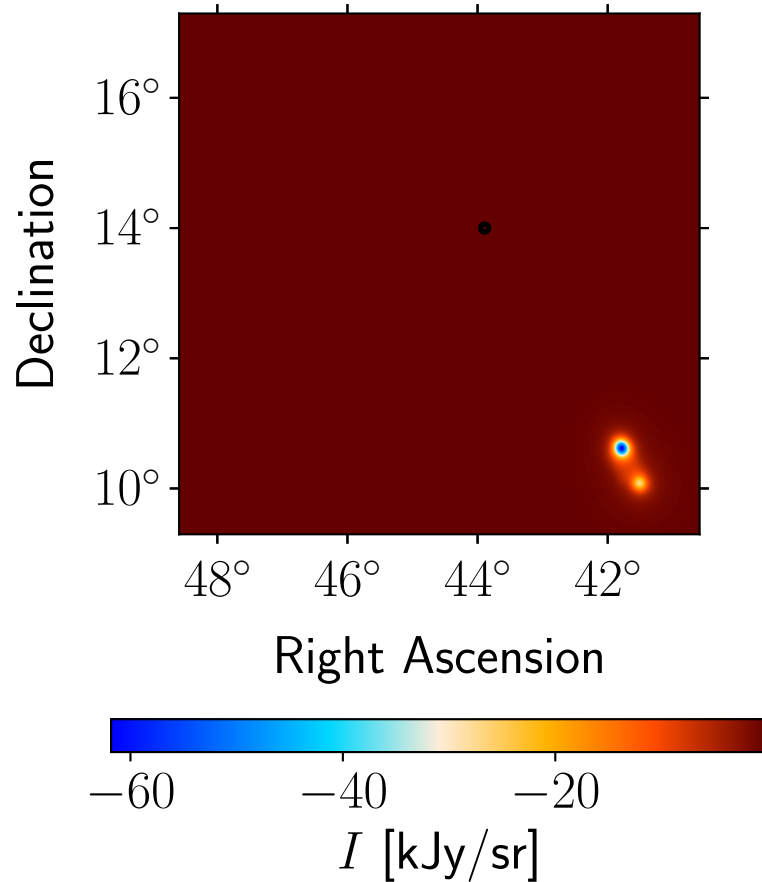
Model: Planck 143 GHz
