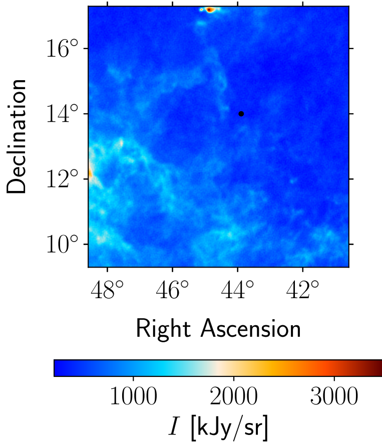
Data: Planck 353 GHz
