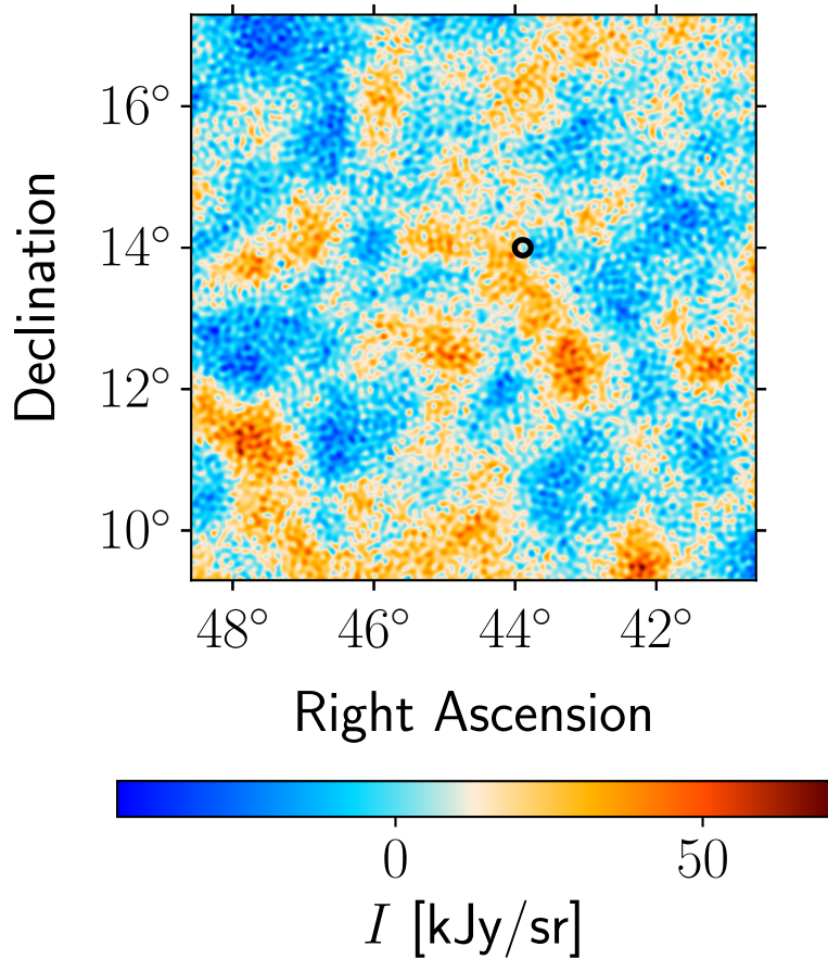
Data: Planck 70 GHz
