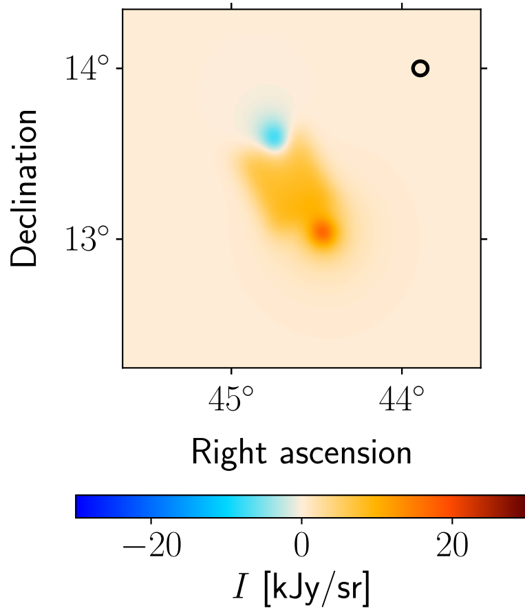
Model: Planck 217 GHz
