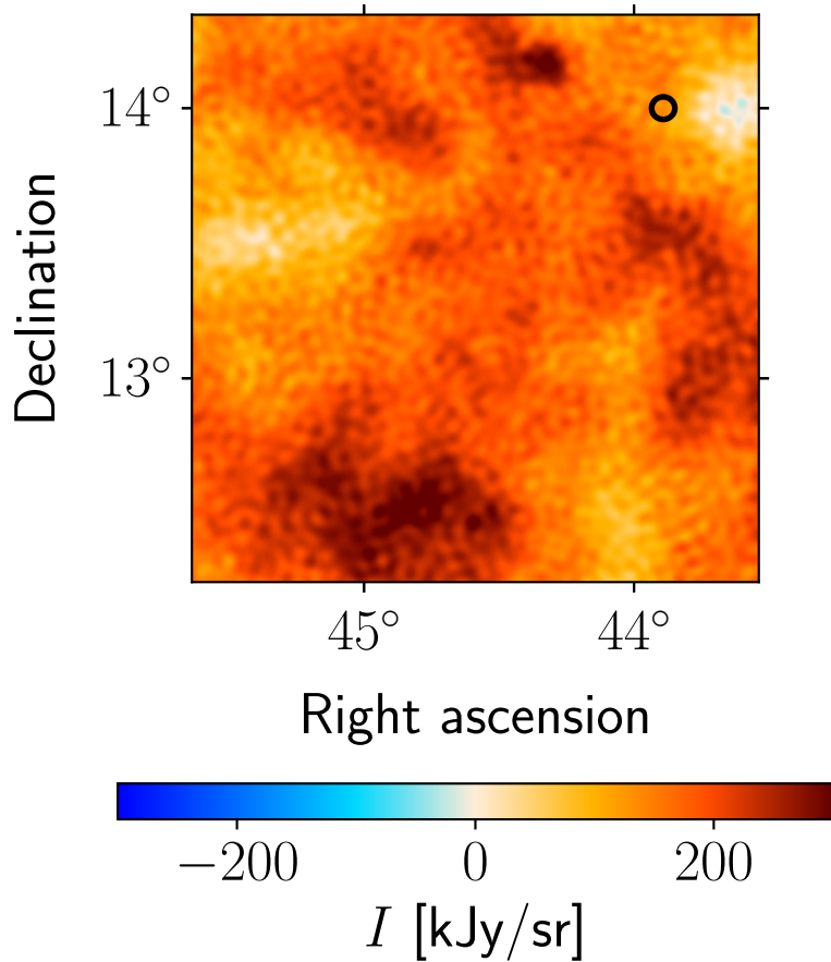
Data: Planck 217 GHz
