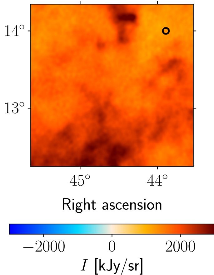
Data: Planck 545 GHz
