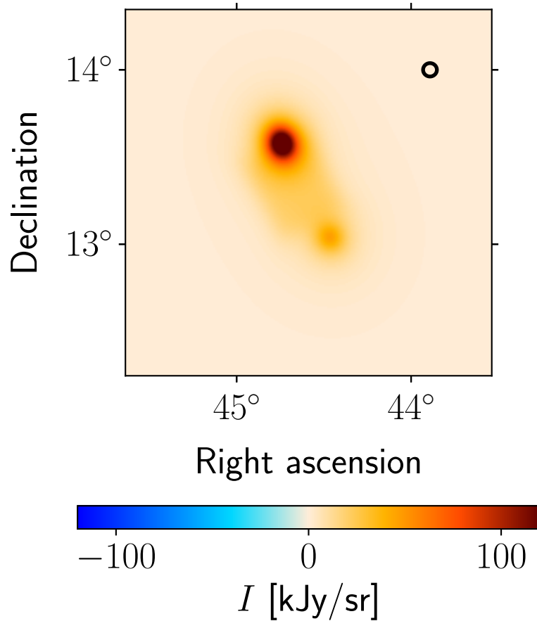
Model: Planck 545 GHz
